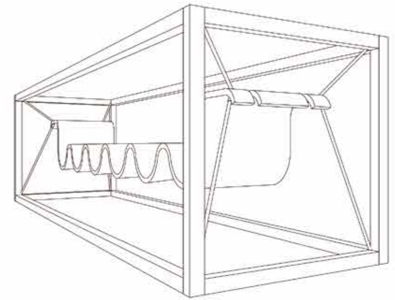
PROSPETTIVA
